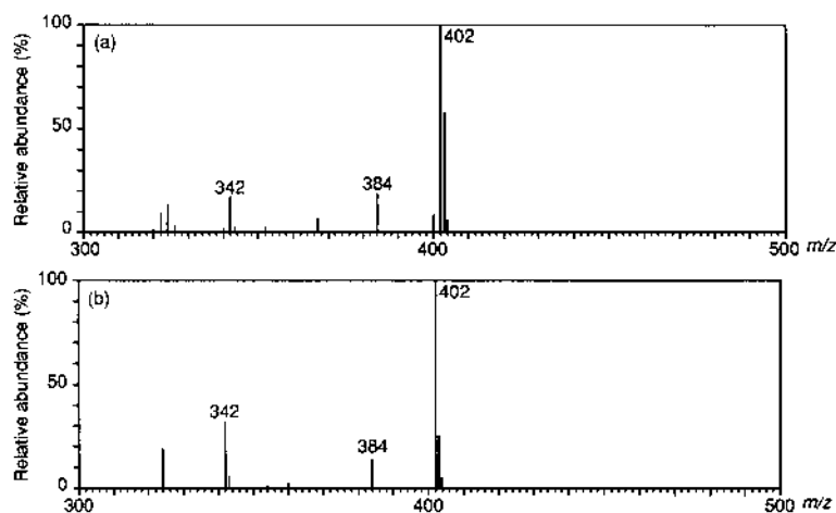
Fig. 7. APCI Mass Spectra of Alkaloids Lucidusculine ( 5 ; a) and 12- Epi -lucidusculine ( 6 ; b)
